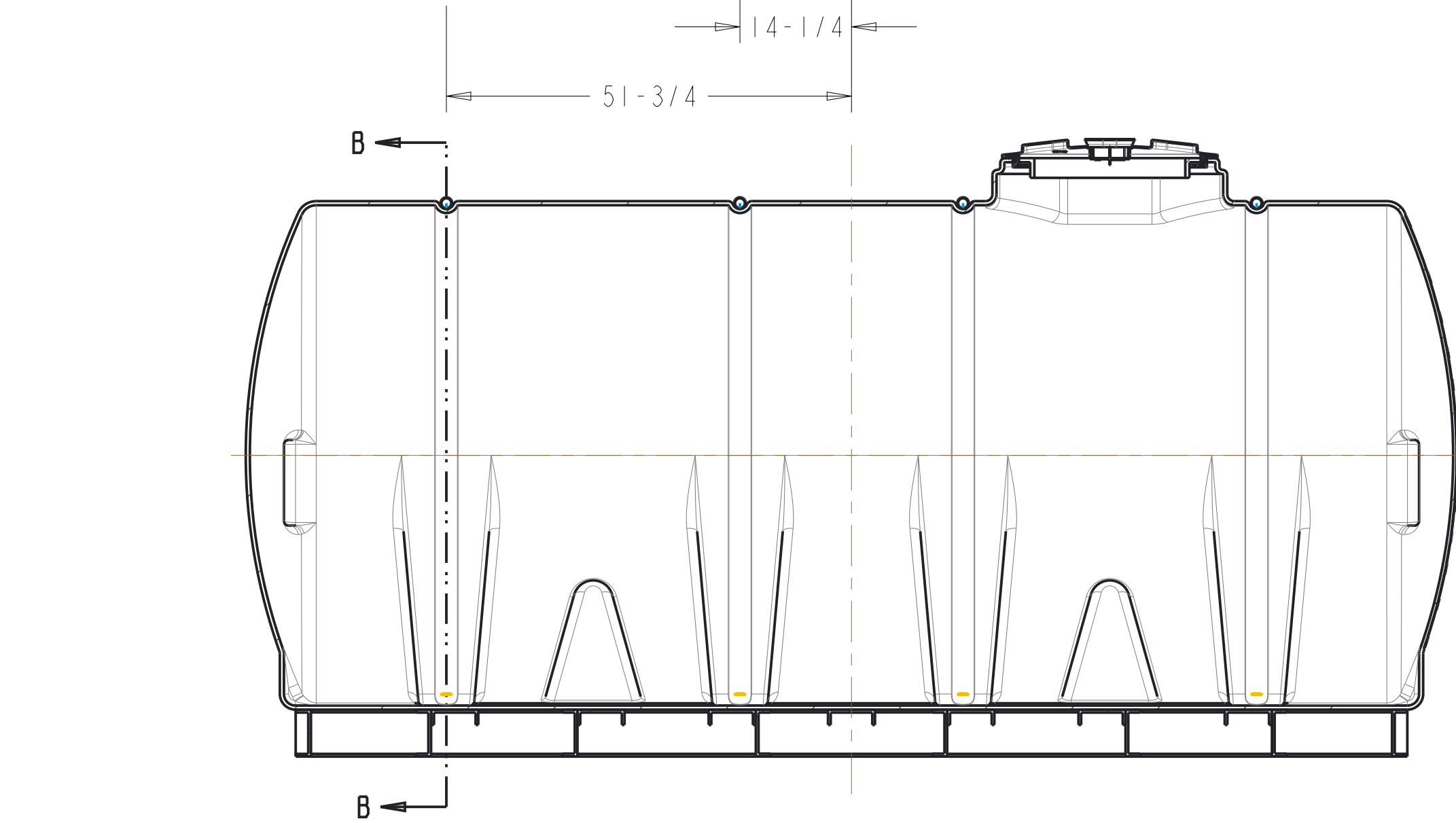
SECCIÓN A-A
